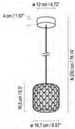
Nans S /16 IP-66
