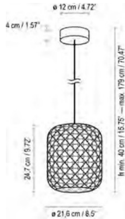
Nans S /21 IP-66
