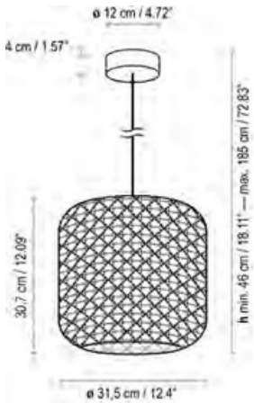
Nans S /31 IP-66
