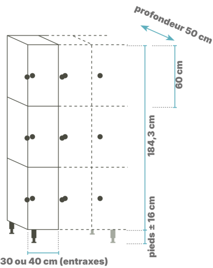
3 CASES PAR COLONNE Réf. : 113.X3
