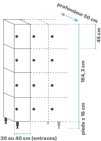
4 CASES PAR COLONNE Réf. : 113.X4
