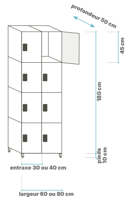
4 CASES PAR COLONNE Réf. 115.114
