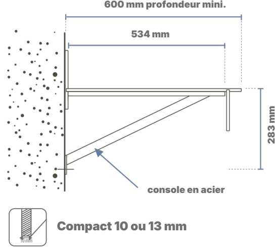
Fixation sur consoles murales
