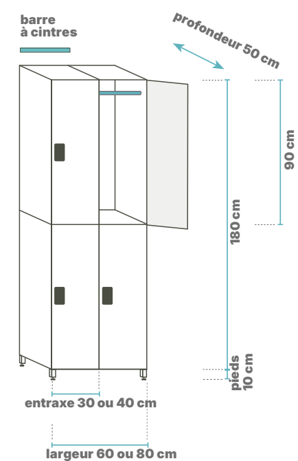
2 CASES PAR COLONNE Réf. 115.112
