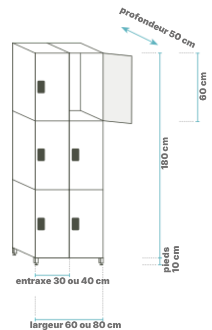
3 CASES PAR COLONNE Réf. 115.113
