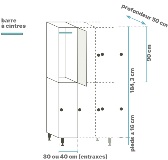
2 CASES PAR COLONNE Réf. : 113.X2
