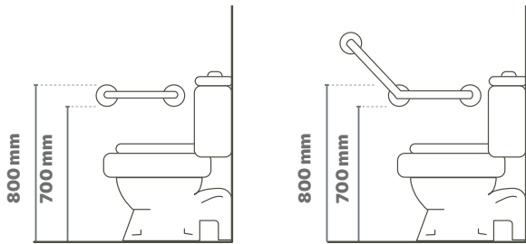
Barre de relevage droite Barre de relevage coudée
