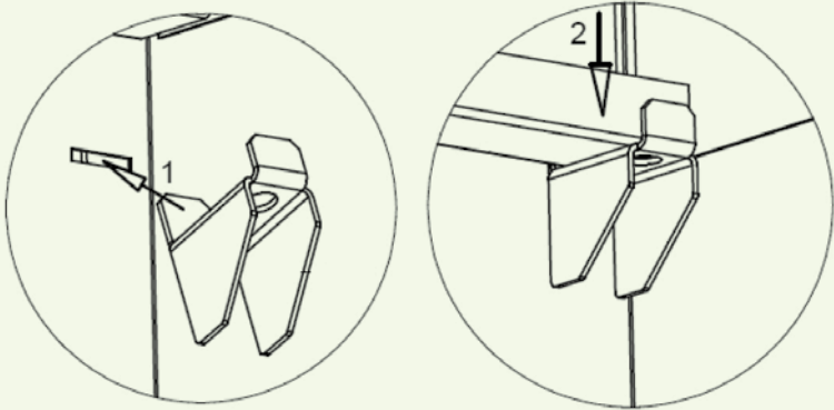
Sposób montażu zaczepów do półki.
