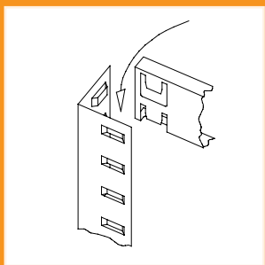
system montażu regałów „na wcisk”
