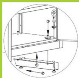
stopki poziomujące - sposób regulacji
